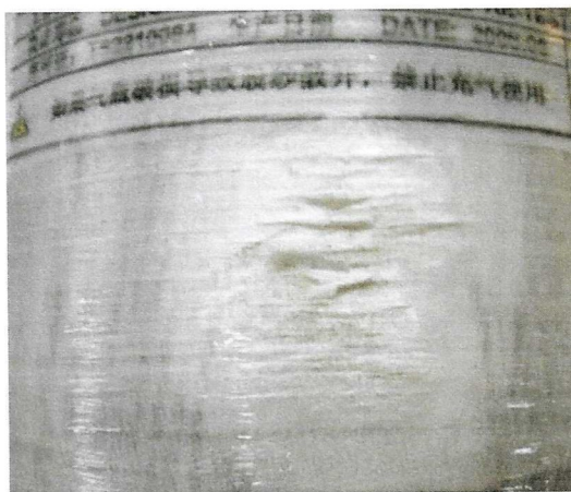
图 B.9 冲击损伤(二级损伤)
