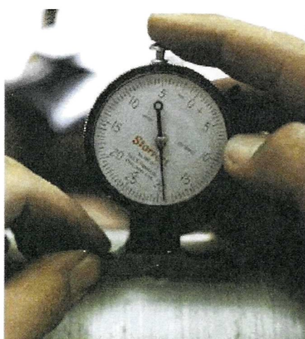
图 C.2 深度测量
