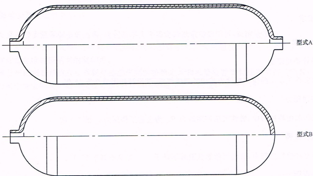
图 1 结构型式
