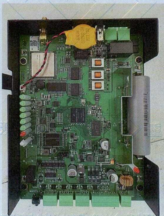
TD-LTE 无线数据终端内部结构图
