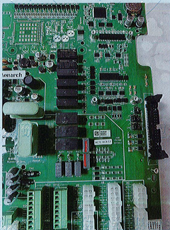
电梯控制装置 (MCTC-MCB-E3)
