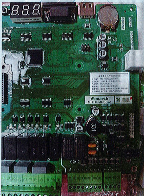
电梯控制装置 (MCTC-MCB-C2)
