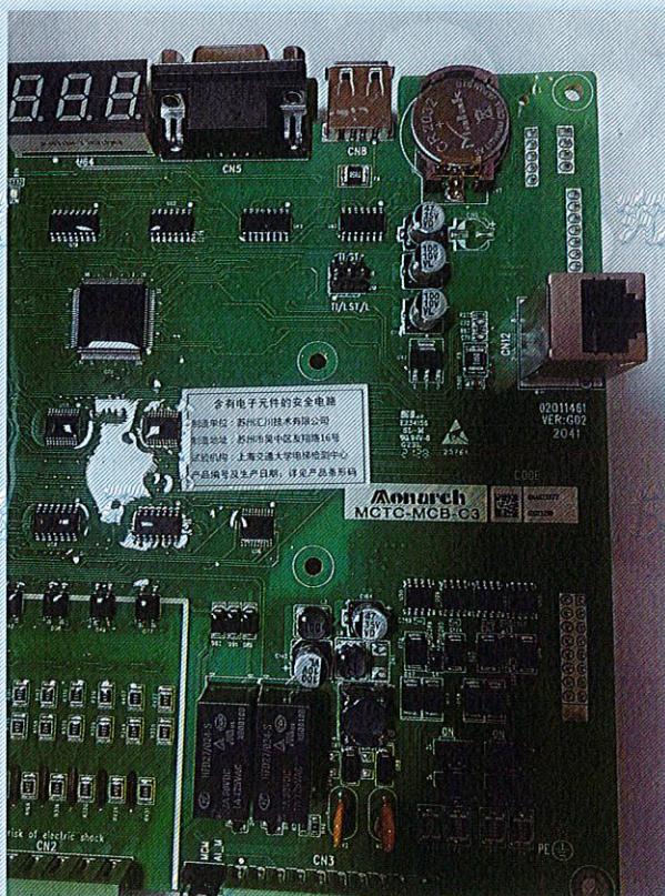
电梯控制装置 (MCTC-MCB-C3)
