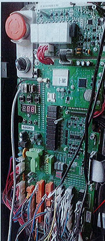
电梯控制装置 (GM90-MCB-Q3)
