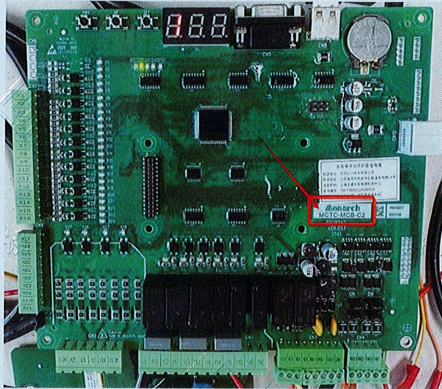
电梯控制装置 (MCTC-MCB-C2)
