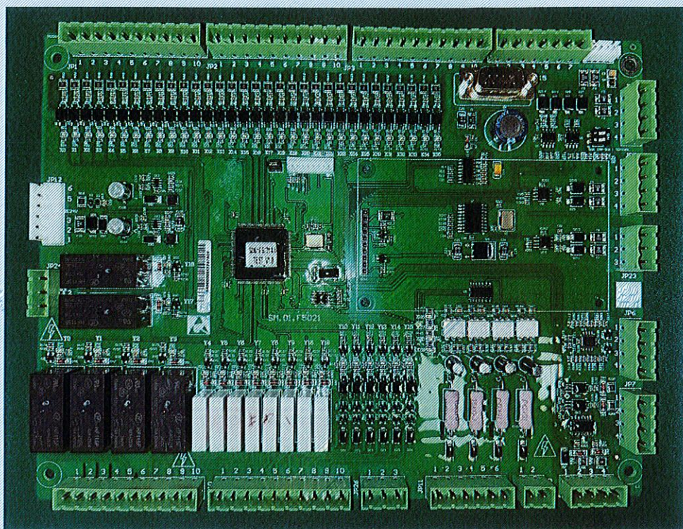
电梯控制装置(SM.01.F5021)
