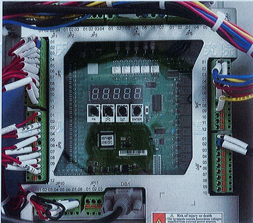
电梯控制装置(AS.T029)
