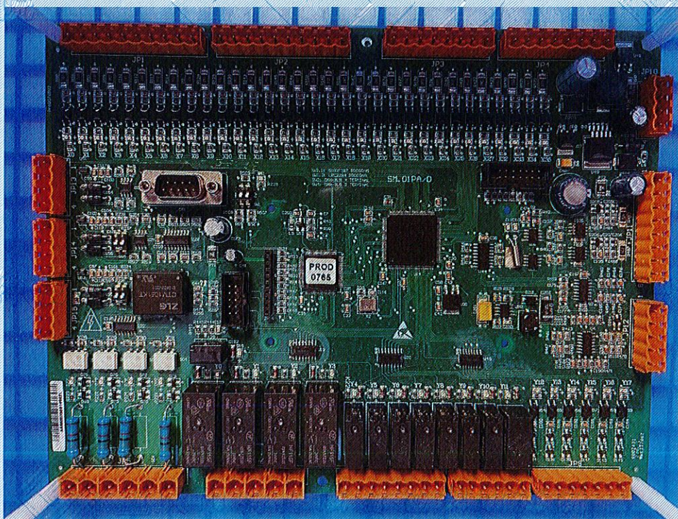
电梯控制装置 (SM.01PA/D)
