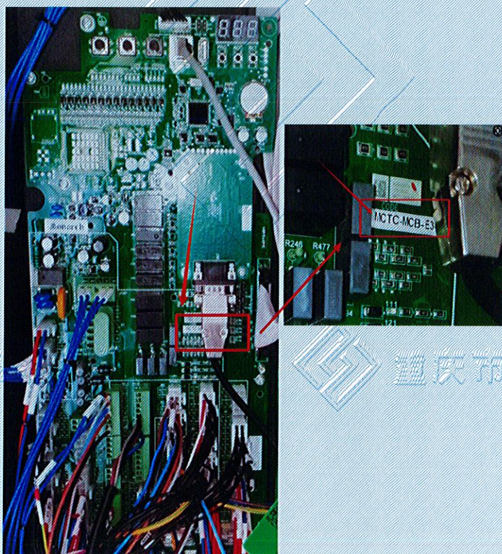
直梯控制装置 (MCTC-MCB-E3)
