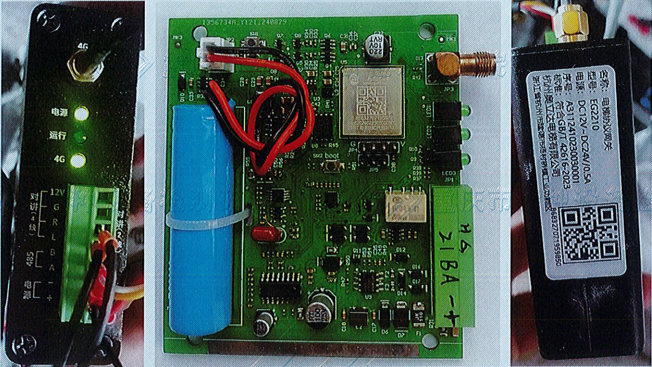
电梯协议网关 (EG2210)
