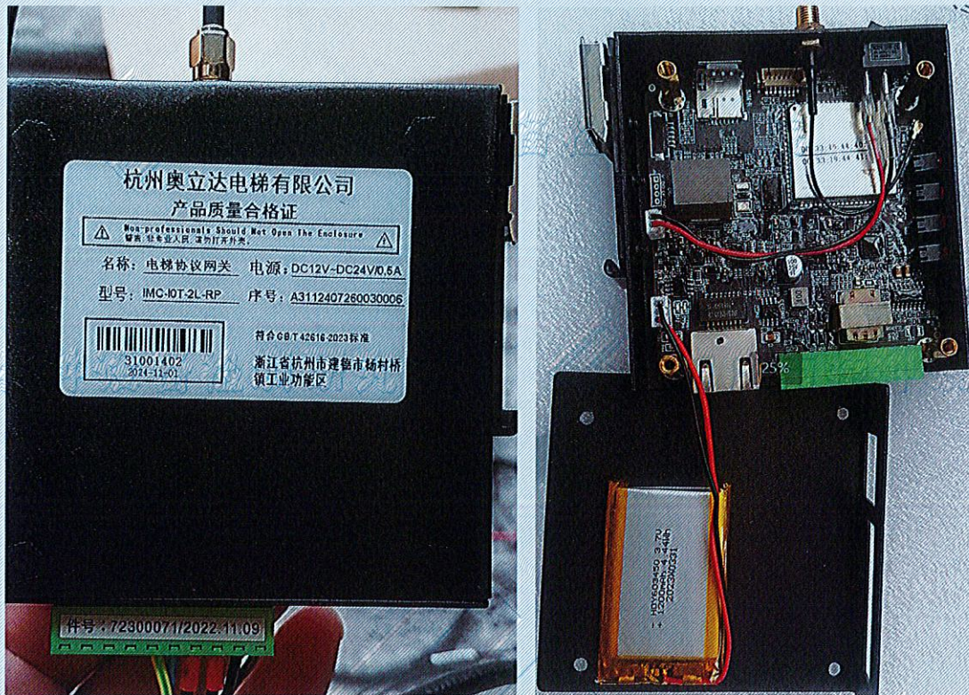
电梯协议网关 (IMC-IOT-2L-RP)
