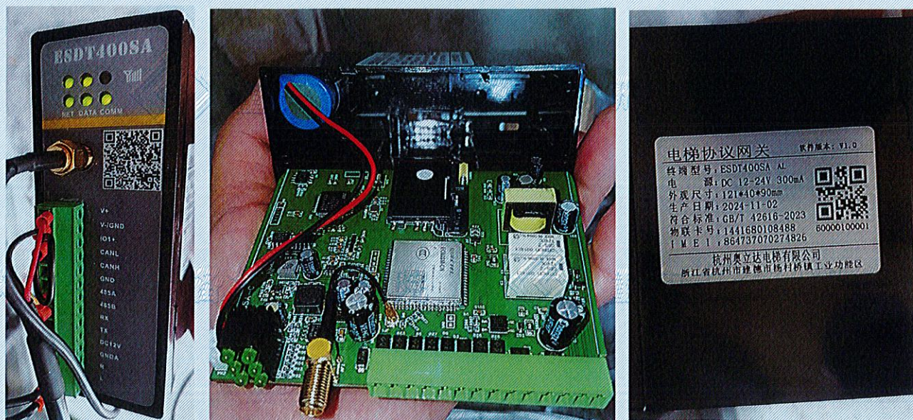
电梯协议网关 (ESDT400SA AL)
