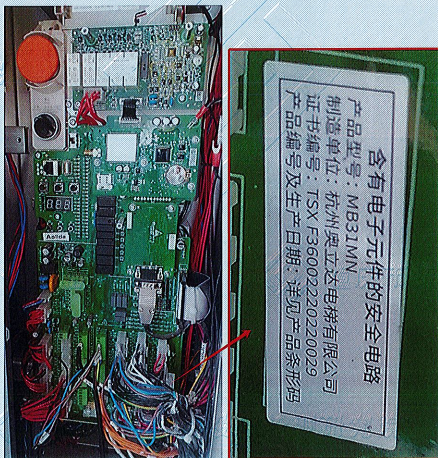
电梯控制装置 (MB31MN)
