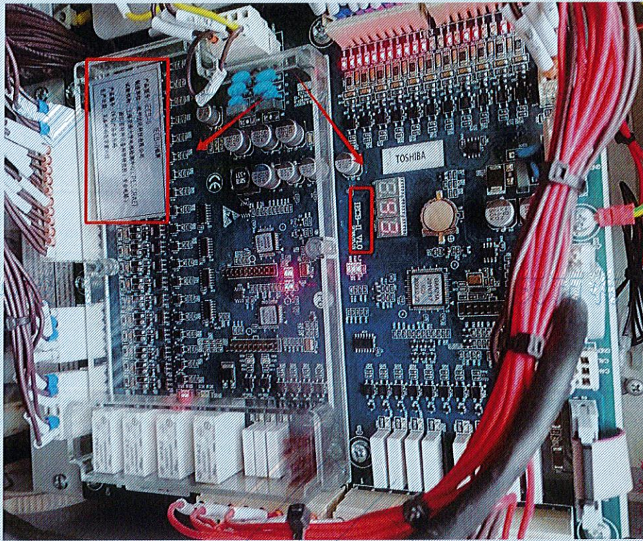
扶梯/人行道控制装置 (IECB-II)
