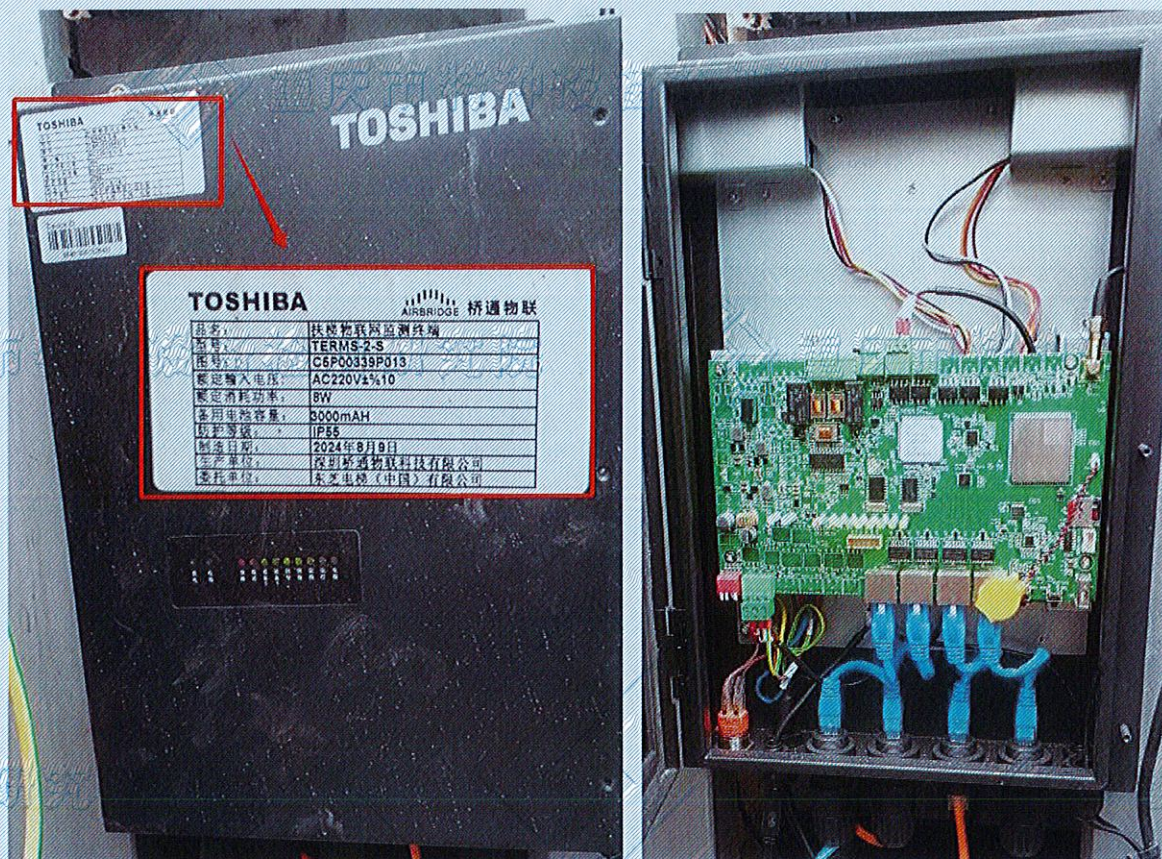
扶梯物联网监测终端 (TERMS-2-S)
