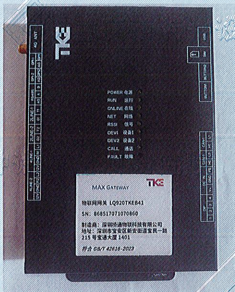
物联网网关及电源适配器
