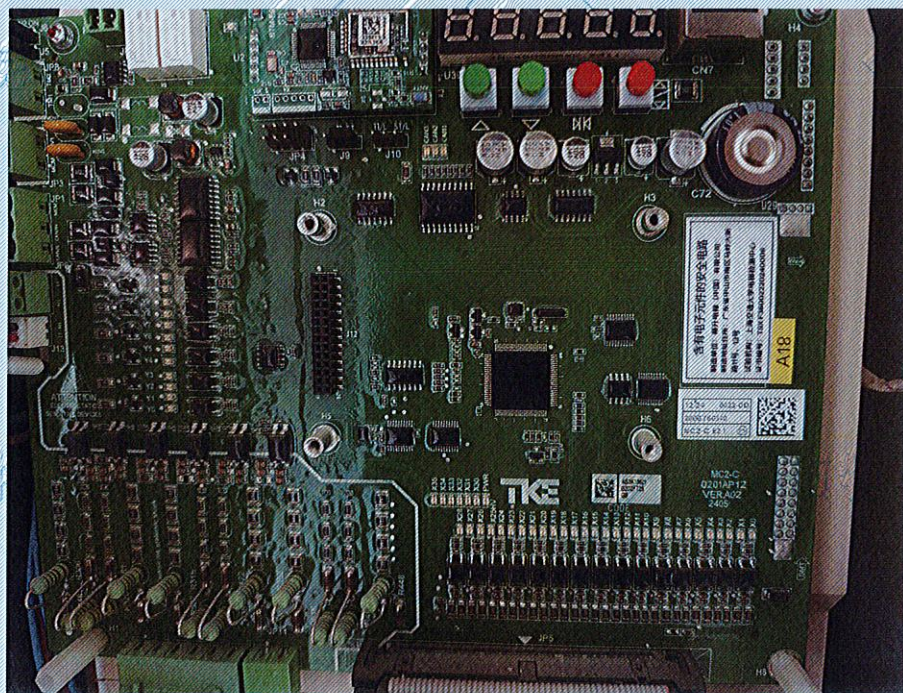
电梯控制装置(MC2-C)
