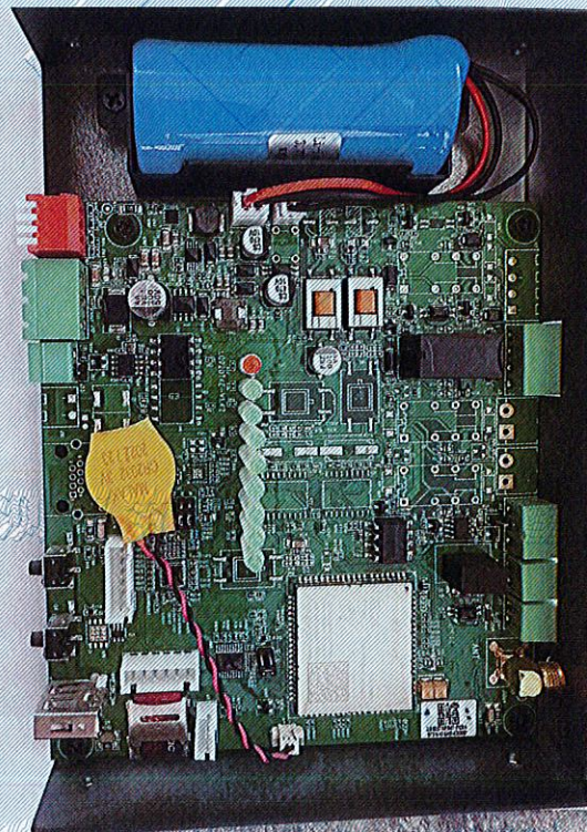
物联网网关内部结构图
